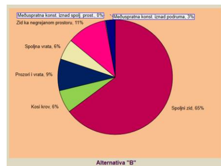
Slika 3. Transmisioni gubici sklopova i njihov udeo u ukupnim gubicima omotača, alternativa „B“.
