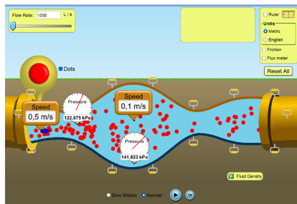
Слика 2. Изглед Phet симулације протока флуида [4].
