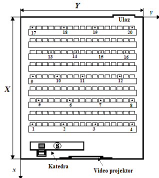
Slika 1. Prikaz amfiteatra u kome je izvršen eksperiment: S - lokacija zvučnog izvora, 1 – 20 – lokacija prijemnika.
