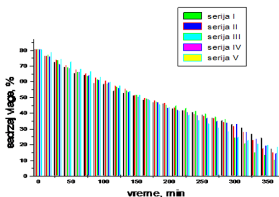
Slika 1. Dijagram promene sadržaja vlage tokom vremena sušenja sveže višnje bez tretmana, (serija I), tretirane vitaminom C, (serija II), limontusom, (serija III), vinobranom (serija IV) i glinom (serija V).
