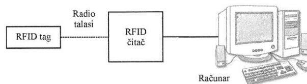
Slika 5. RFID sistem
