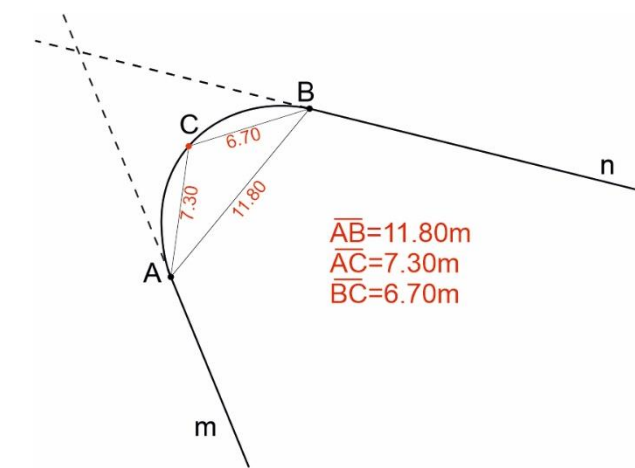
Slika 2-A. Postupak merenja krivine.
