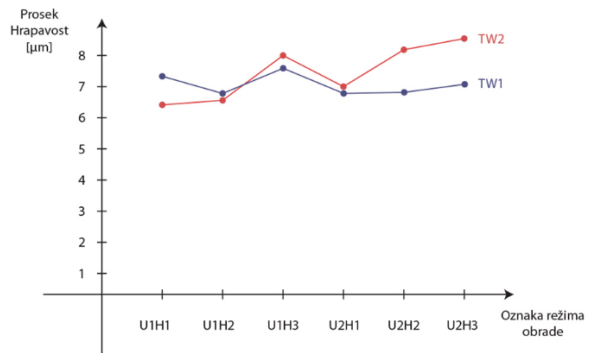
Slika 6. Kretanje srednje vrednosti hrapavosti u zavisnosti od režima obrade.
