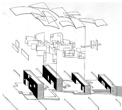
Slika 11. Eksplodiran aksonometrijski prikaz kuće
