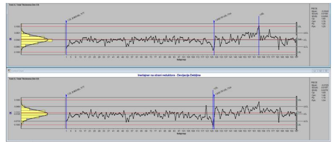
Slika 3. Kontrolni dijagram.
