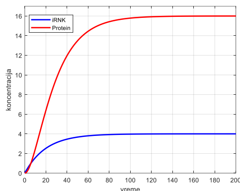
Slika 2. Dinamika koncentracije iRNK i proteina tokom vremena.
