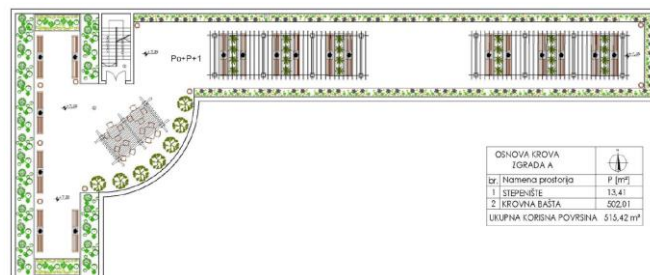
Slika 4. Idejno rešenje osnove krovne bašte zgrade kolektivnog stanovanja.
