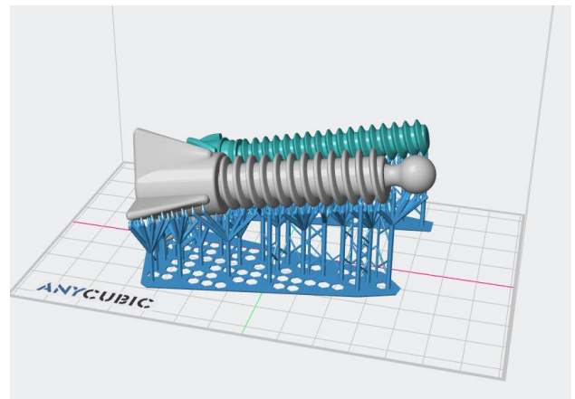
Slika 2. Prikaz delova u softveru PhotonWorkshop.
