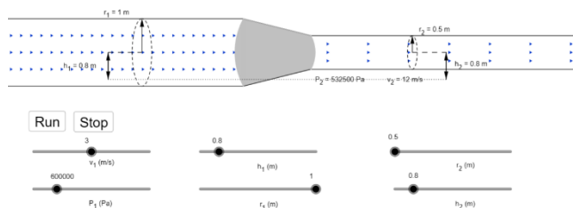
Слика 1. Изглед ophysics симулације протока флуида [3].
