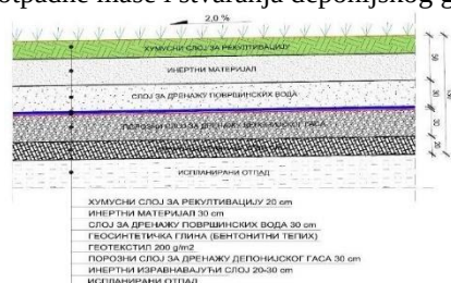
Slika 2. Slojevi zatvaranja spoljašnjih površina tela deponije.
