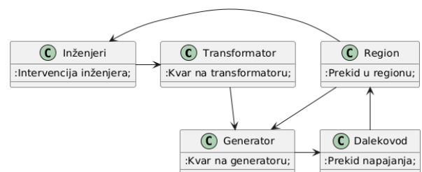
Slika 3. CLD kreiran pomoću rezultata primene LLM-a. Dijagram koristi JSON podatke i prikazuje kako greške u jednom procesu mogu izazvati lančanu reakciju u sistemu.
