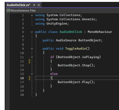
Slika 10. C# kod za pokretanje audio zapisa klikom na dugme.
