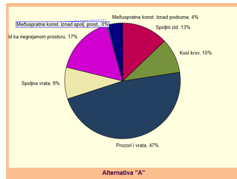
Slika 2. Transmisioni gubici sklopova i njihov udeo u ukupnim gubicima omotača, alternativa „A“.
