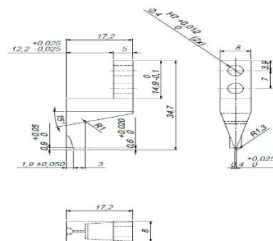
Slika 5. Dimenzije alata.
