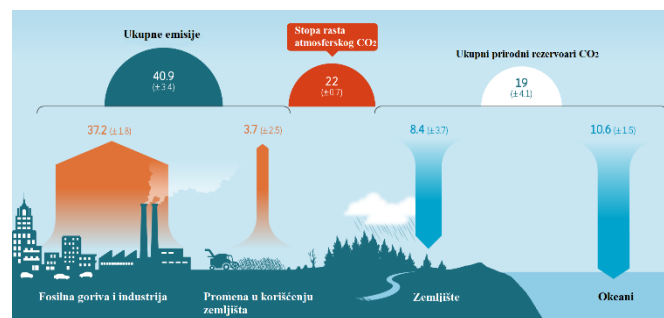
Slika 1. Globalni budžet za \text{CO}_2 za 2023. godinu [9]
