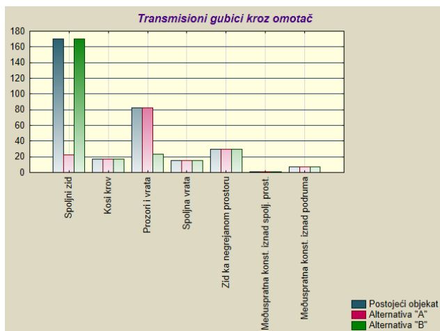
Slika 4. Uporedni prikaz transmisivnih gubitaka sklopova i njihov udeo u ukupnim gubicima omotača.
